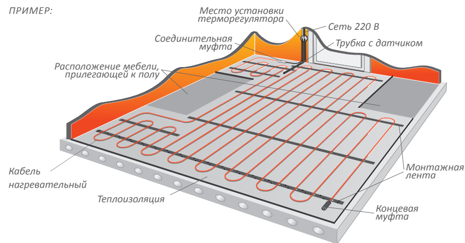
Схема раскладки двужильного нагревательного кабеля
