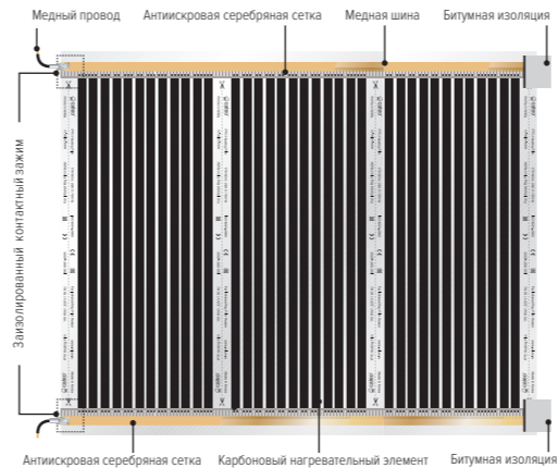
Рис. Общий вид термоленты CALEO, расположение основных ее элементов, контактных зажимов и мест подключения и изоляции
